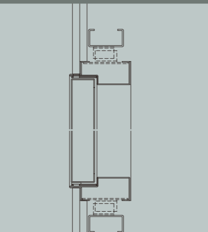
点検口ドアWH断面
