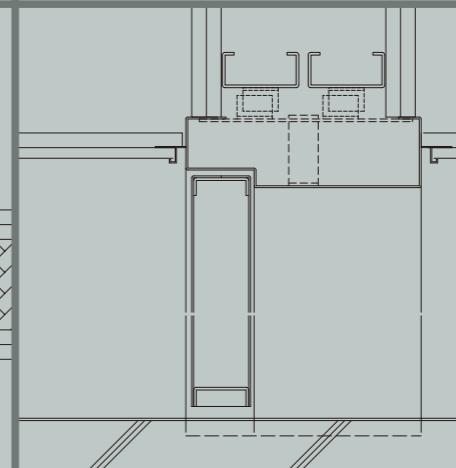
防火ドアH断面【90°開き】
