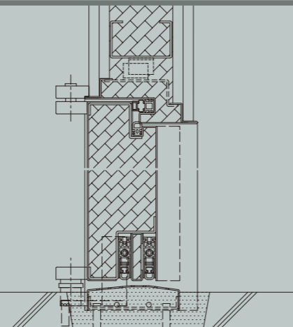
防音ドアWH断面【T-4等級】
