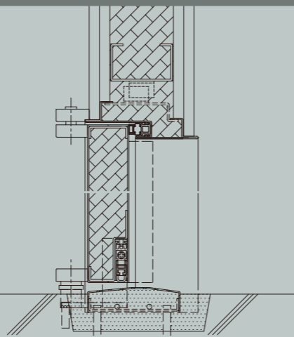
防音ドアWH断面【T-2等級】
