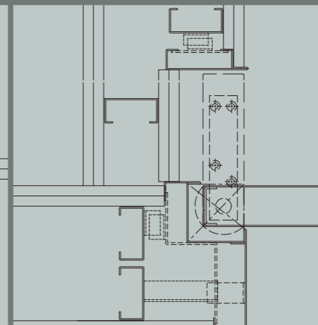
防火ドアW断面【90°開き】
